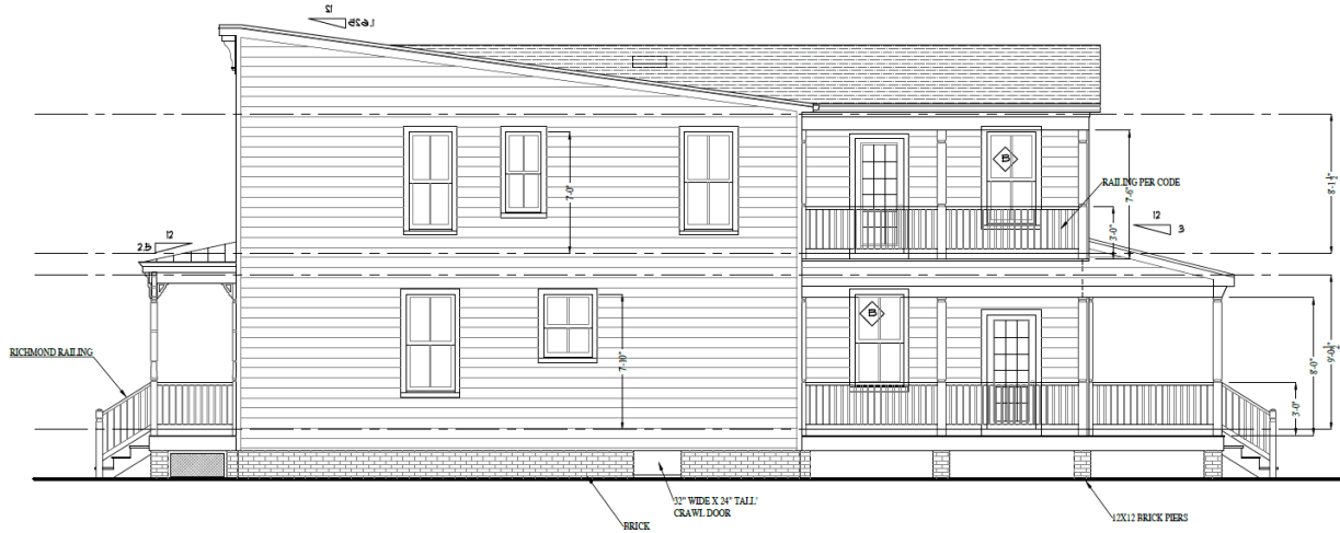
RIGHT ELEVATION
