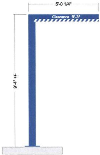
01 ELEVATION
