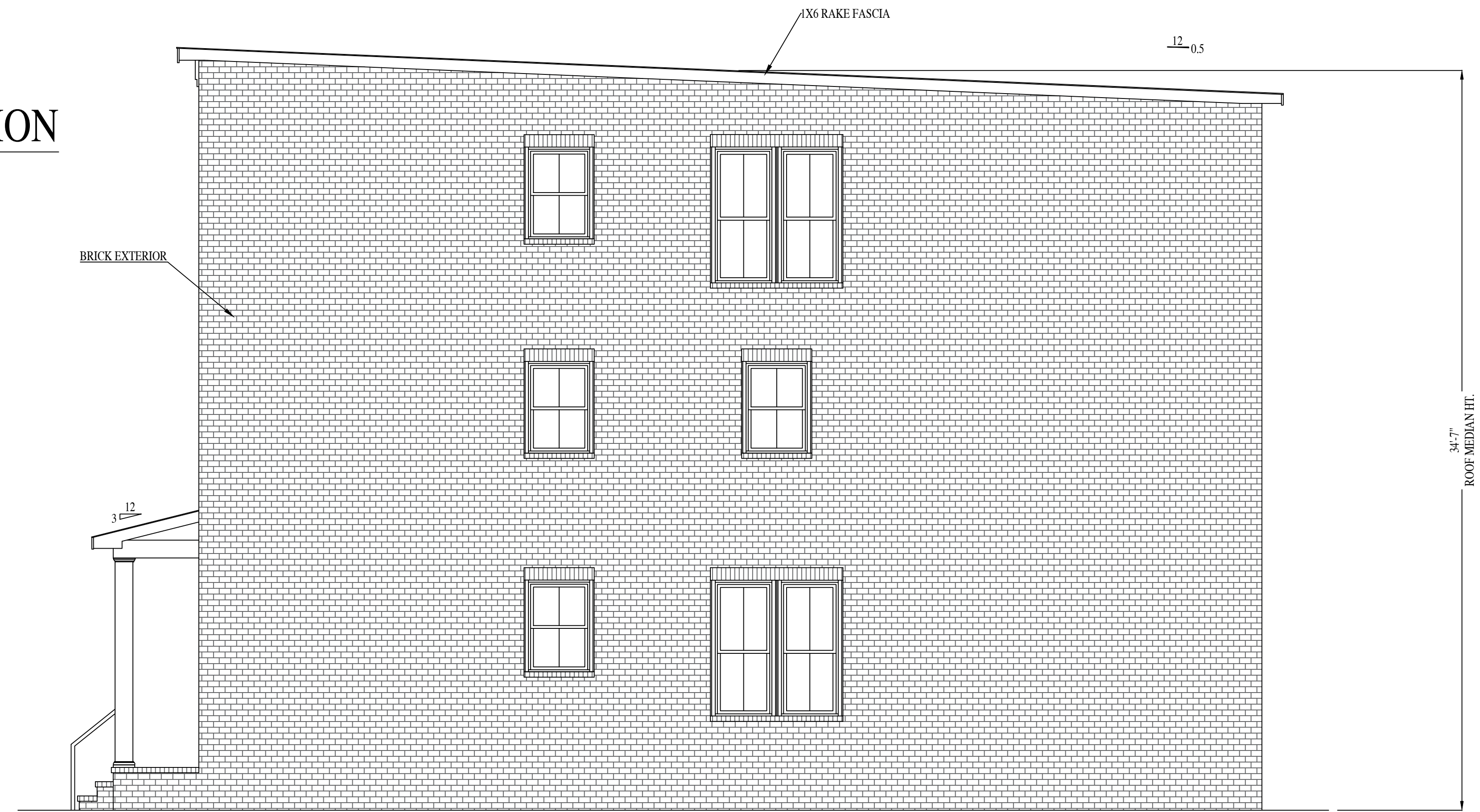
RIGHT ELEVATION
